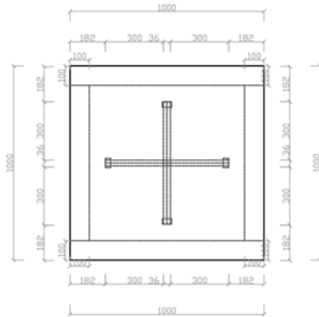
Հատակագիծ
